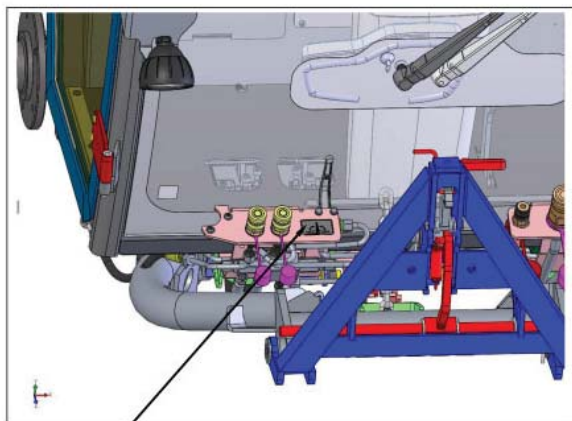
1 17268244 – Druckentlastung
